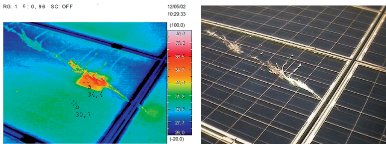
Abb 4.8.11: Zellenüberhitzung durch Verschmutzung, Quelle: L. Erbe
