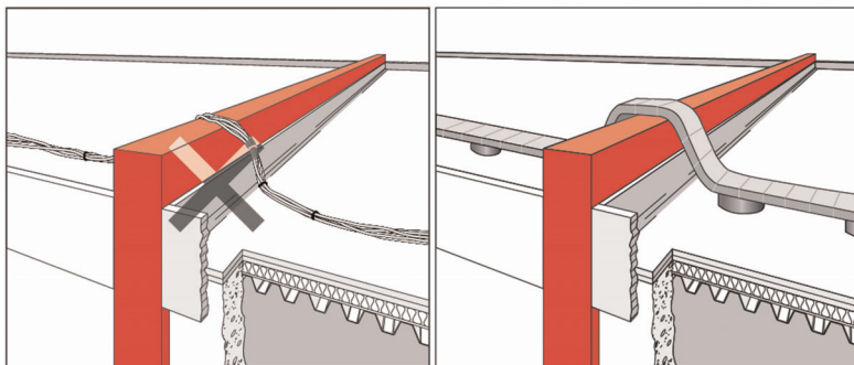
Abb 4.8.4: Kabelführung über eine Brandwand, Quelle: VdS 2234
