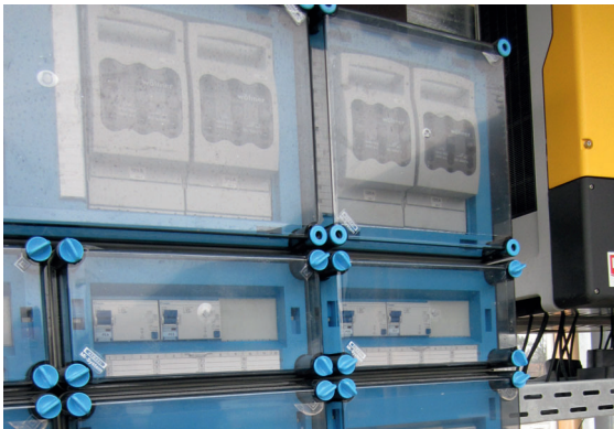
Abb 4.8.9: Wechselrichterverteilung mit RCD, Quelle: VGH Versicherungen
