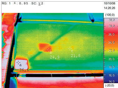
Abb 4.8.12: Hotspot durch Verschattung, Quelle: L. Erbe
