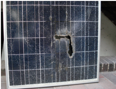
Abb 4.8.13: Lichtbogenschaden am PV-Modul, Quelle: VGH Versicherungen
