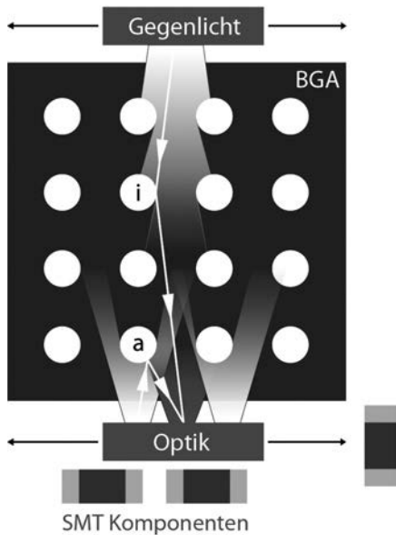
Bild 4.4: Prinzip der BGA-Inspektion – Draufsicht (Quelle: ERSa GmbH)
