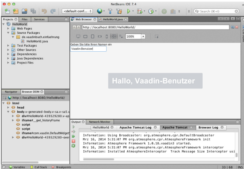
Abb. 2-7 Unsere erste Applikation mit NetBeans
