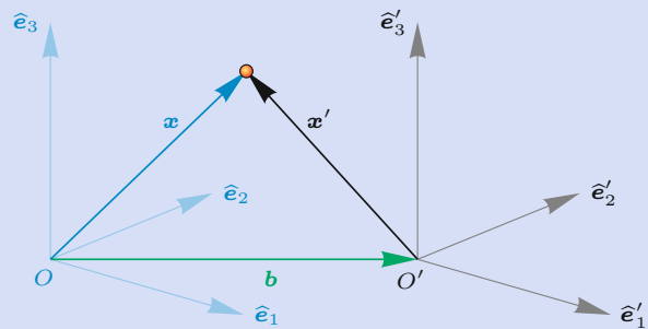
Abb. 2.4 Transformation zwischen kartesischen Koordinatensystemen. Der Ursprung des gestrichenen Koordinatensystems S' befindet sich vom ungestrichenen Koordinatensystem S aus betrachtet am Ort \boldsymbol{b} . Eine Punktmasse hat in S die Ortskoordinaten \boldsymbol{x} (blau), in S' \boldsymbol{x}' (schwarz)
