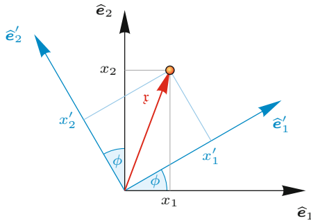
Abb. 2.3 Darstellung einer passiven Drehung, bei der das ungestrichelte Koordinatensystem (schwarz) durch eine Drehung um die x_3 -Achse in das gestrichelte Koordinatensystem (blau) überführt wird. Der Vektor \boldsymbol{x} wird davon nicht berührt, allerdings hängt seine Darstellung vom Koordinatensystem ab, wie man an den Projektionen auf die entsprechenden Koordinatenachsen erkennen kann
