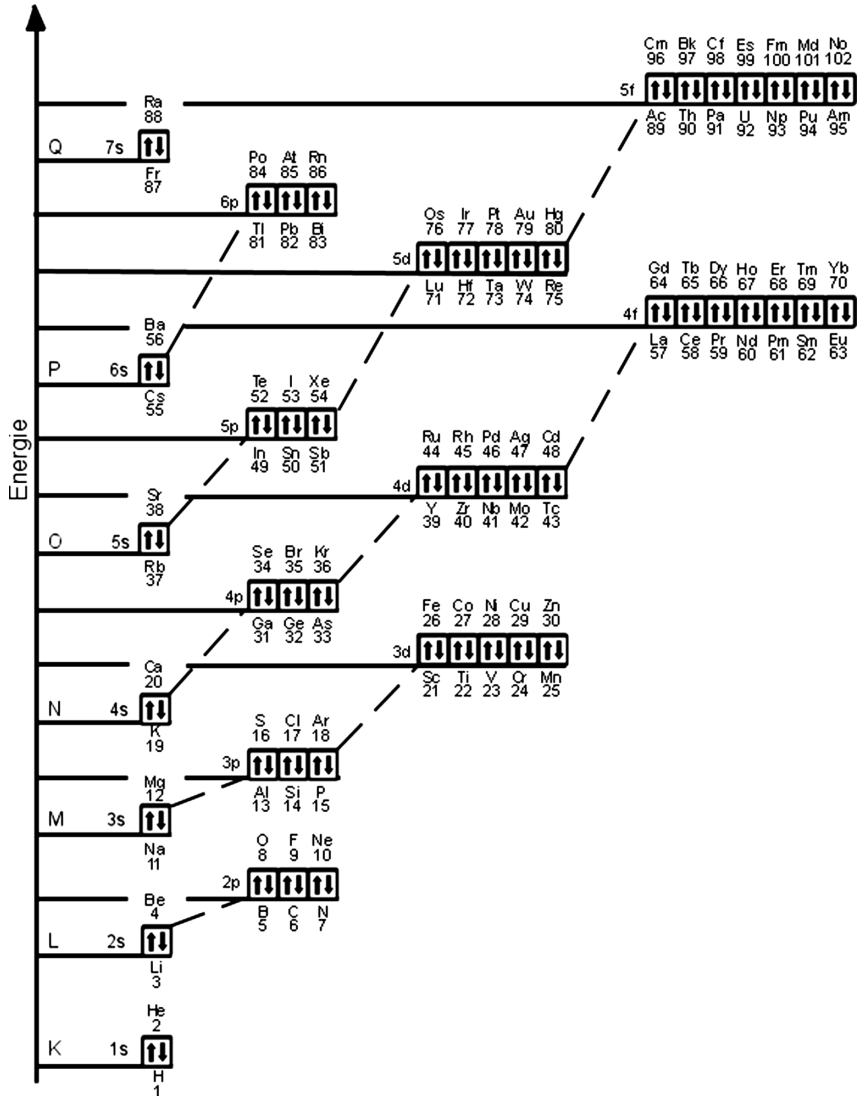
Abb. 1.6 Energieniveauschema.
