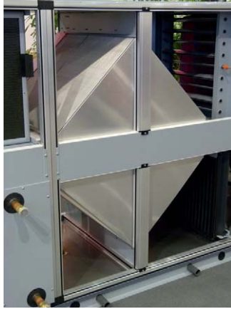
Abb. 2.1 Einsatz eines Kreuzstromwärmeübertragers in einem RLT-Gerät (Quelle: M. Stahl)
