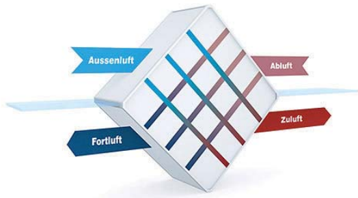
Abb. 2.4 Prinzipielle Darstellung der Wärmeübertragung in einem Kreuzstromwärmeübertrager (Quelle: Klingenburg GmbH)
