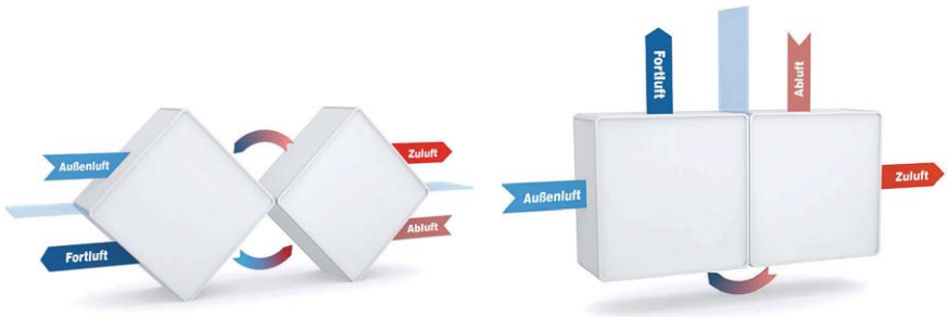
Abb. 2.8 und 2.9 Kopplung von zwei Kreuzstromwärmeübertragern in diagonaler Ausführung (links) und in einer Reihenordnung (rechts). (Quelle: Klingenburg GmbH)
