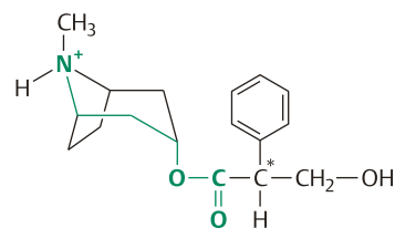
Atropin *asymmetrisches Kohlenstoffatom
