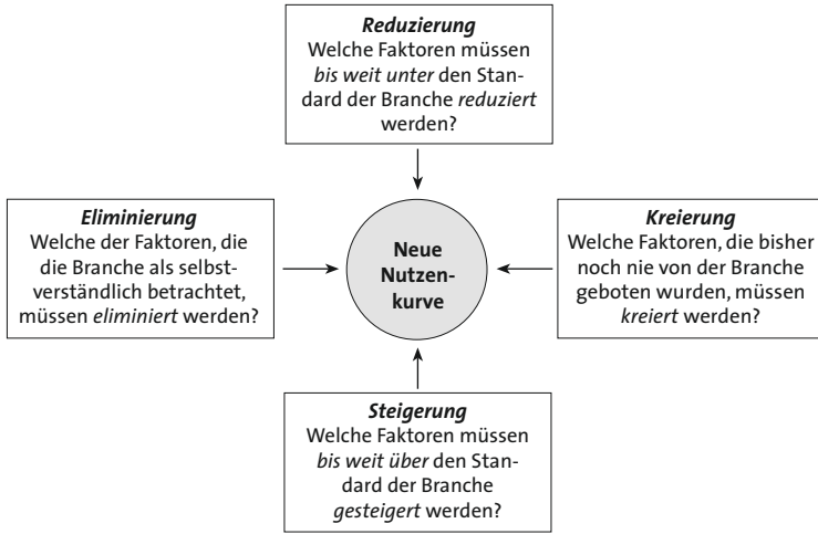
Abb. 2.2: Das Vier-Aktionen-Format
