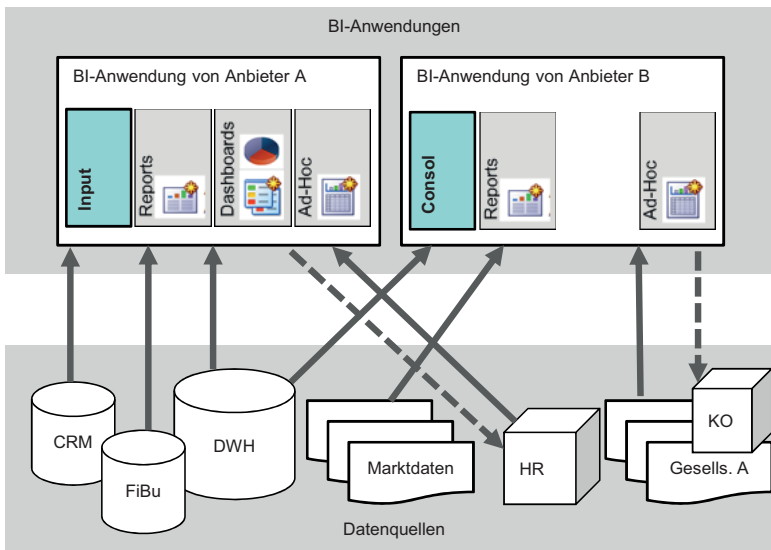
Bild 2.5 BI-Anwendungen/BI-Tools teilen Datenquellen und Funktionalitäten.
