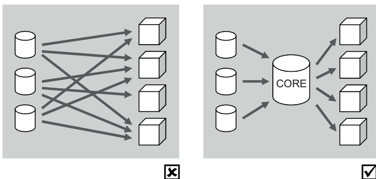
Bild 2.3 ETL-Prozesse mit und ohne Core
