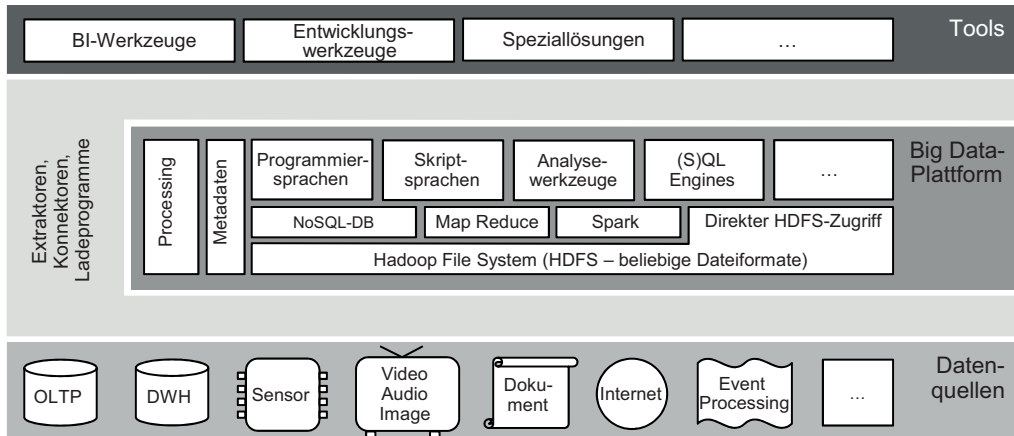
Bild 2.8 Datenhaltung und Verarbeitung mittels Big Data-Technologien aus Sicht des Hadoop-Ecosystems
