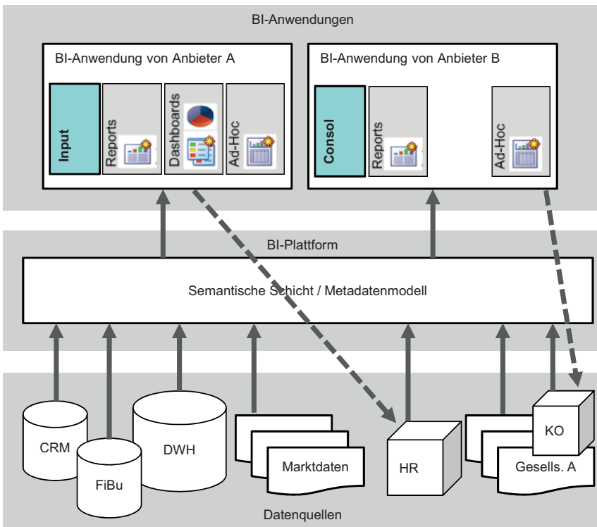
Bild 2.6 Die BI-Plattform als Schnittstelle zwischen BI-Anwendungen/BI-Tools und Data Warehouse und weiteren Datenquellen
