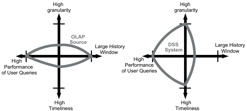
Bild 2.4 Unterschiedliche Anforderungen an Data Marts
