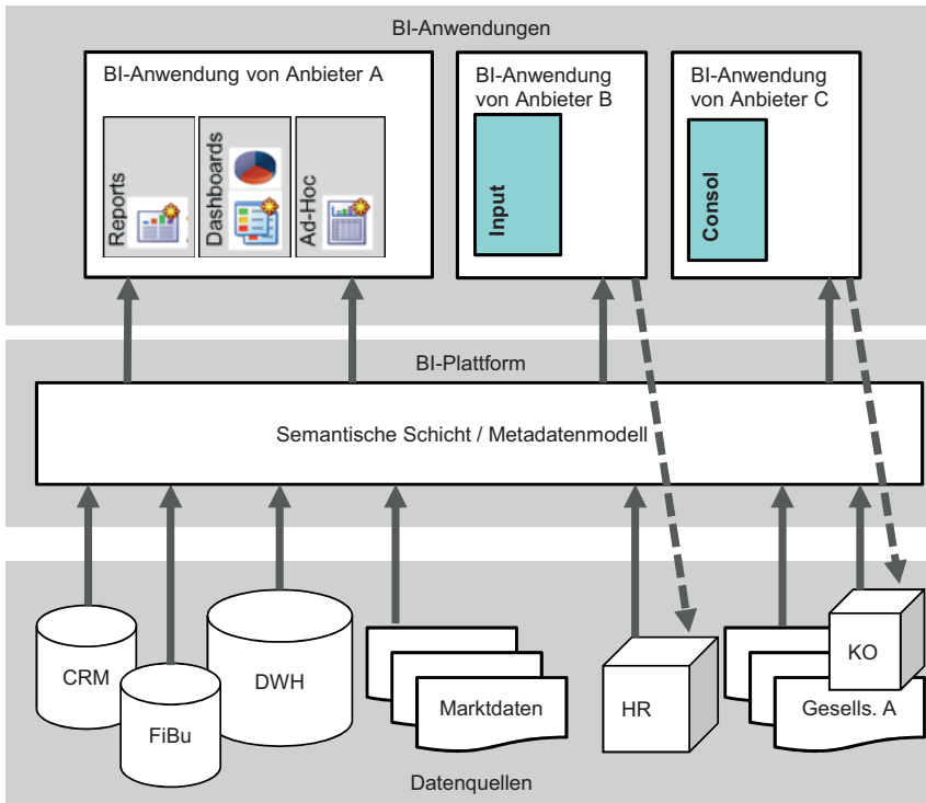
Bild 2.7 Die BI-Plattform als Schnittstelle zwischen BI-Anwendungen und Datenquellen
