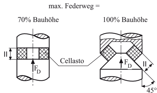
Bild 4.24: Erhöhung des Federweges einer Elastomer-Feder gleicher Bauhöhe durch Änderung der Beanspruchungsrichtung
