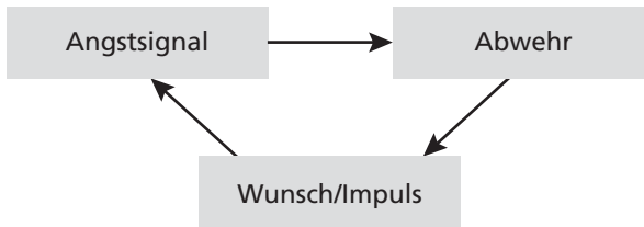
Abb. 1: Konflikt-Dreieck
