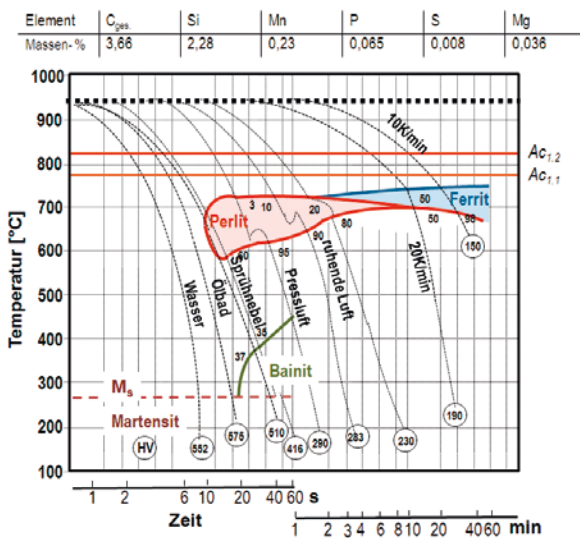
Abb. 5.24: Kontinuierliches Zeit-Temperatur-Umwandlungsschaubild (ZTU) für unlegiertes Gusseisen mit Kugelgraphit (Austenitisierungstemperatur 950 °C, Kugelzahl ca. 500 m 2 ): Abhängig von den Abschreckbedingungen erzielte Härte (HV) (nach Herfurth 1971, Davis 1996)
