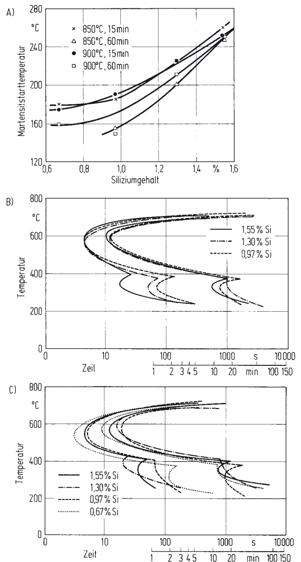
Abb. 5.31: Einfluss unterschiedlicher Siliziumgehalte auf die Umwandlung von schwarzem Temperguss (Siepmann 1970): A) Änderung der Martensitstarttemperatur, B) Umwandlungsbeginn und Umwandlungsende ( T_A: 850\text{ °C} , t_A: 60\text{ min} )
