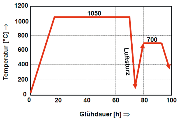
Abb. 5.20: Perlitglühen von weißem Tempereguss GJMW 450-7 (nach Hasse 2008)
