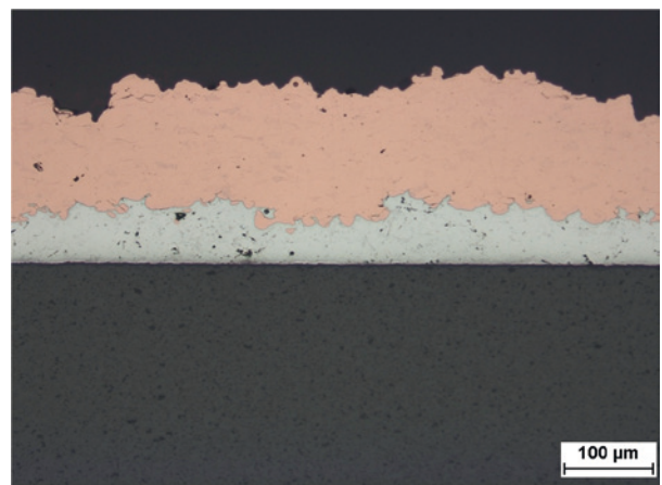
Abb. 4.59: Querschliff einer kaltgasgespritzten Cu-Schicht mit Al-Zwischenlage
