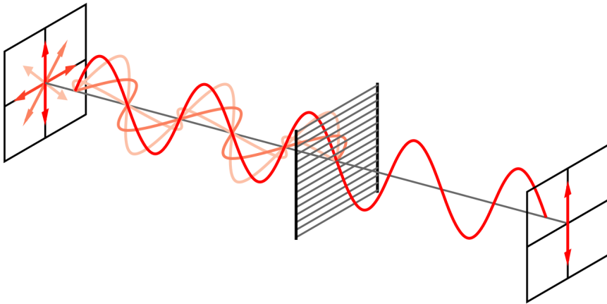
Funktionsprinzip des Polfilters (Quelle: Wikipedia)
