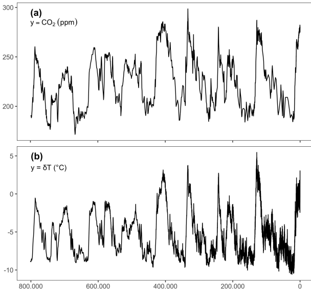
Abb.1: Kohlendioxid- und Temperaturschwankungen in den letzten 800 000 Jahren: (a) Kohlendioxid ( \text{CO}_2 ) in der Atmosphäre in parts per million (ppm). (b) Temperaturschwankungen: Abweichung ( \delta T ) in ^{\circ}\text{C} vom Mittel der letzten 1000 Jahre.
